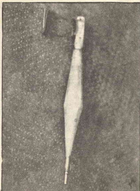
Foto 4. - Tipo di scarico accordato pronto per il montaggio. A sinistra, in basso, il cavallotto d'attacco ricavato da filo d'acciaio armonico da 1 m/m.
