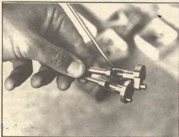
Foto 3. - La foto evidenzia la valvola rotativa e il materiale da asportare onde rendere la luce perfettamente rettangolare. In alto, un albero ancora da elaborare; sotto, una luce finita.
